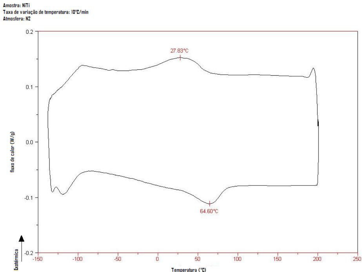
Figura 3: DSC da amostra injetada.
